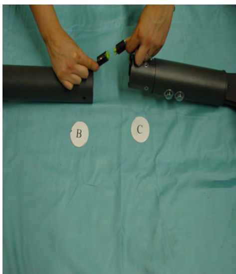
6. Connettere la parte alta del Fungo con i due riscaldatori. Collegare i 2 connettori, far rientrare il cavo connesso nel tubo e infilare i due pali B e C uno nell'altro. Avvitare le 4 viti a brugola da 6MA puntandole prima e poi serrandole. A questo punto l'apparecchio è pronto per essere utilizzato.
